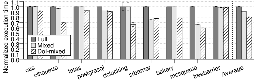
(A) Micro-benchmarks
