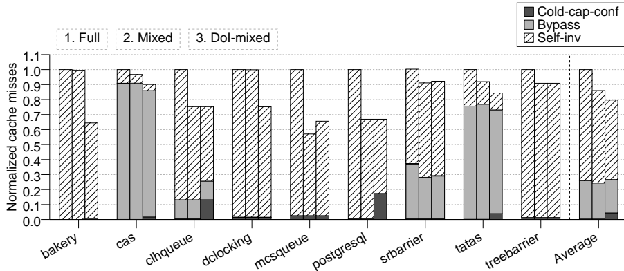
(A) Micro-benchmarks
