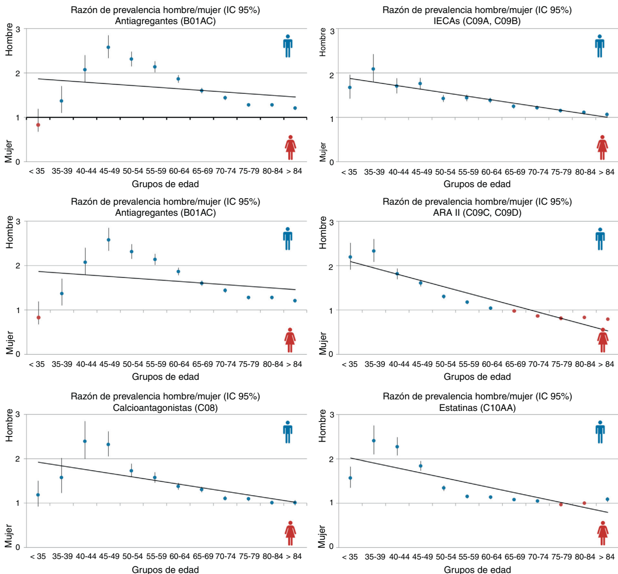
Figura 2 Razones de DHD de medicamentos cardiovasculares por sexo, como cociente de tasas de consumo de hombres respecto a mujeres.
